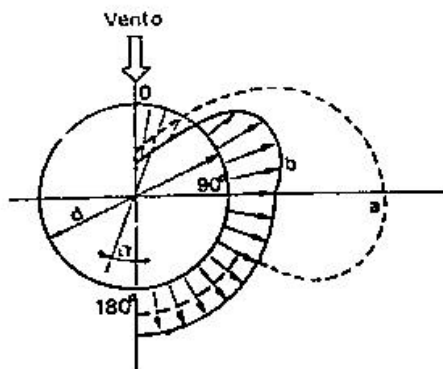
Distribuzione della pressione esterna sulle superfici cilindriche e sferiche
